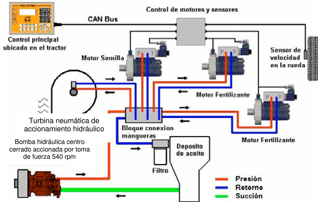
Fig. 1: Esquema del sistema Verión adaptado a una sembradora Agrometal Mega.
